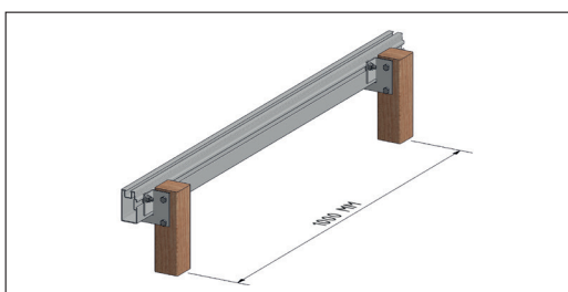
Balk hoog 40 x 75 mm hart op hart afstand 1.000 mm
