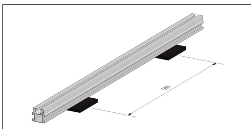
Balk midden 40 x 40 mm hart op hart afstand 500 mm
