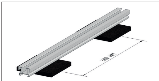
Balk laag 35 x 23 mm hart op hart afstand 300 mm
