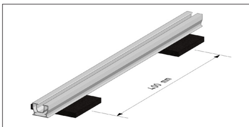
Balk laag 35 x 25 mm hart op hart afstand 400 mm
