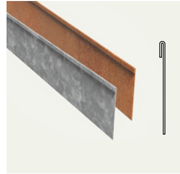
180° DOPPELT GEKANTTET
